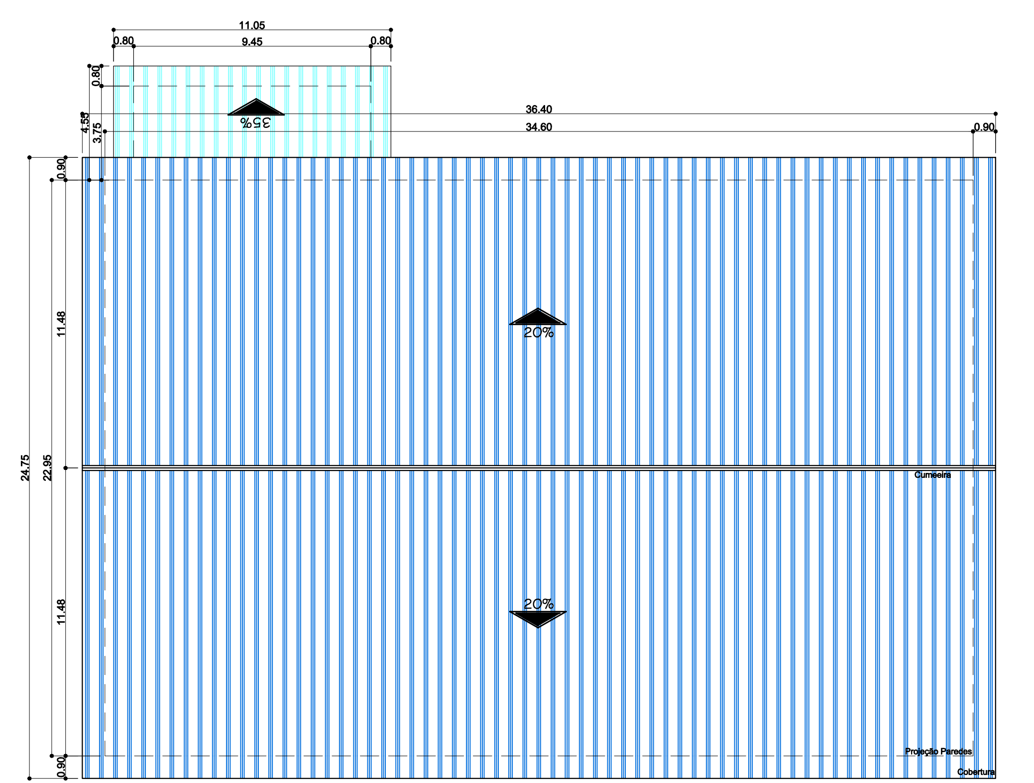
COBERTURA ESCALA ..... 1:150
