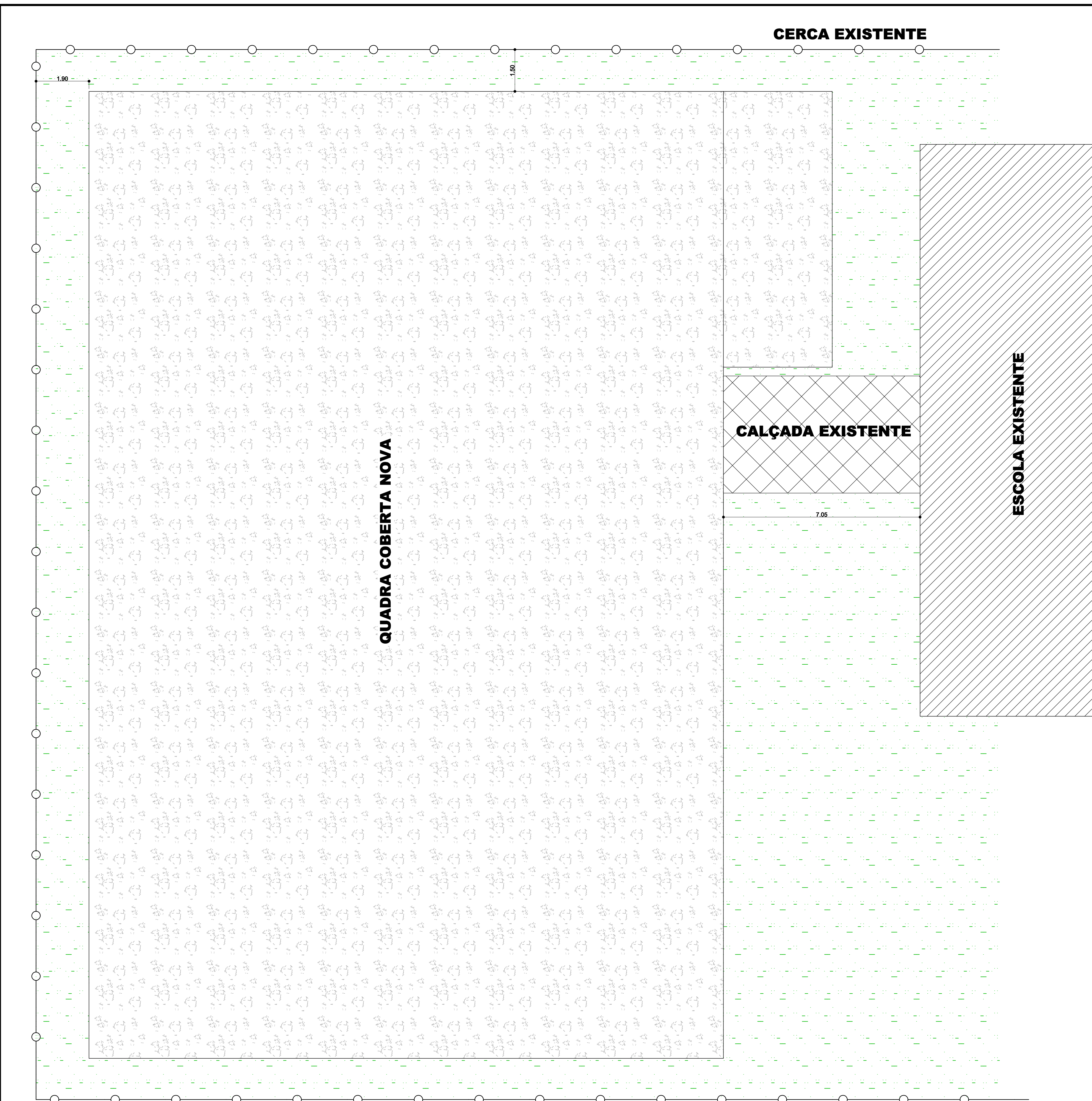
LOCAÇÃO ESCALA ..... 1:75
