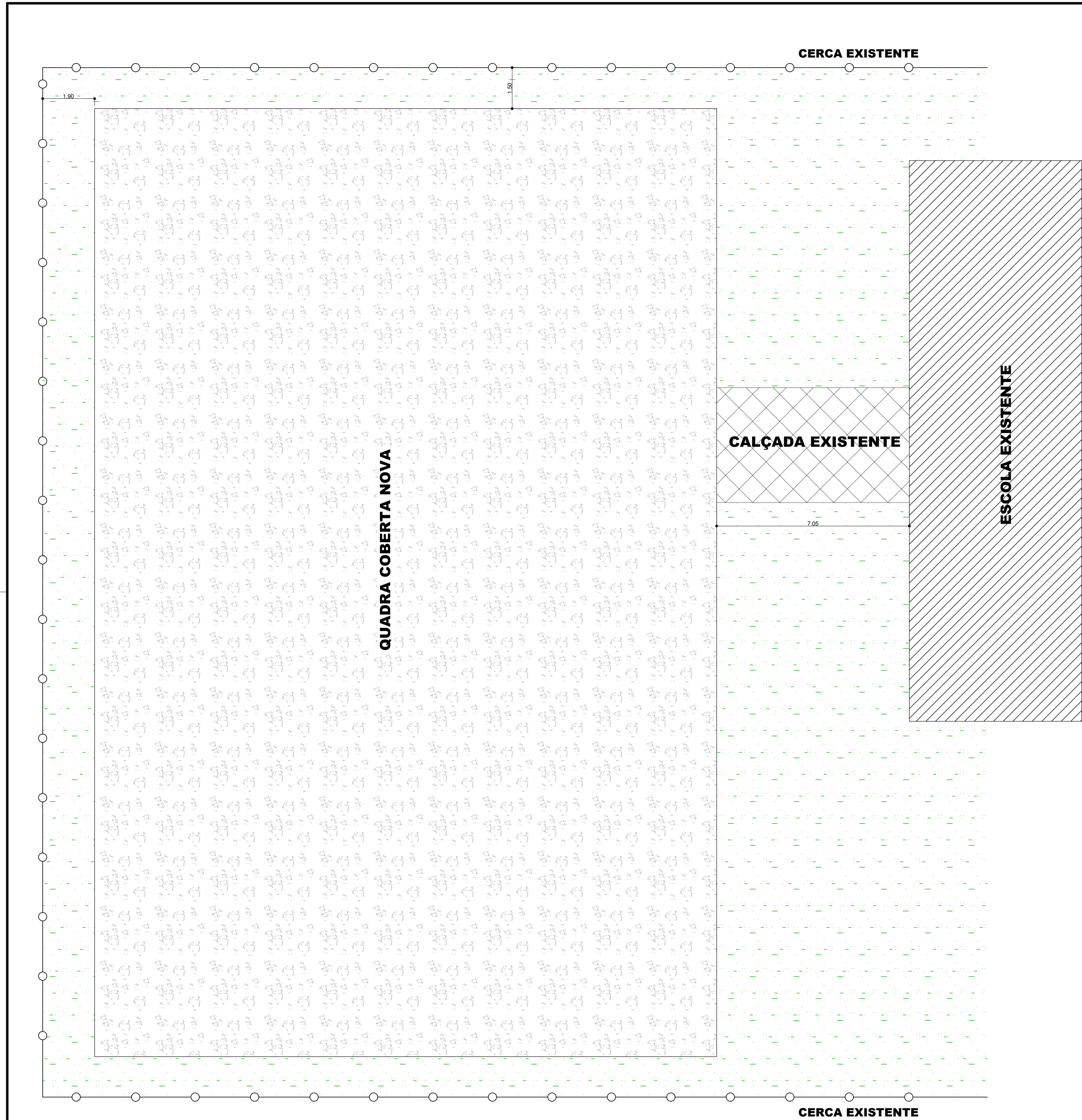
LOCAÇÃO ESCALA ..... 1:75
