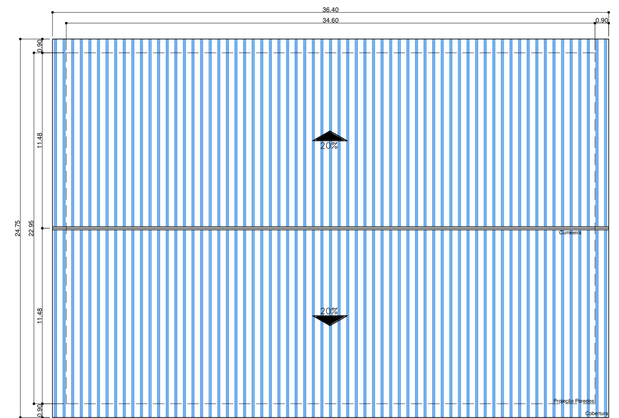
COBERTURA ESCALA ..... 1:150
